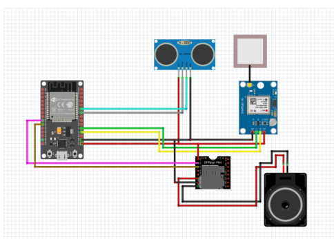
Gambar. 9 Rangkaian Perangkat Keras
