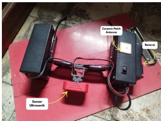
Gambar. 11 Tampak Luar Prototipe Alat Bantu Tunanetra
