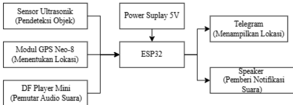
Gambar. 7 Diagram Blok Sistem
