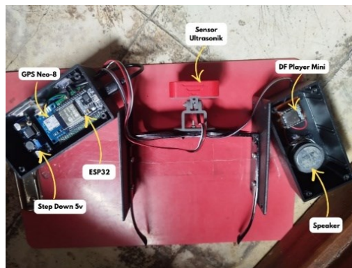
Gambar. 12 Tampak Dalam Prototipe Alat Bantu Tunanetra
